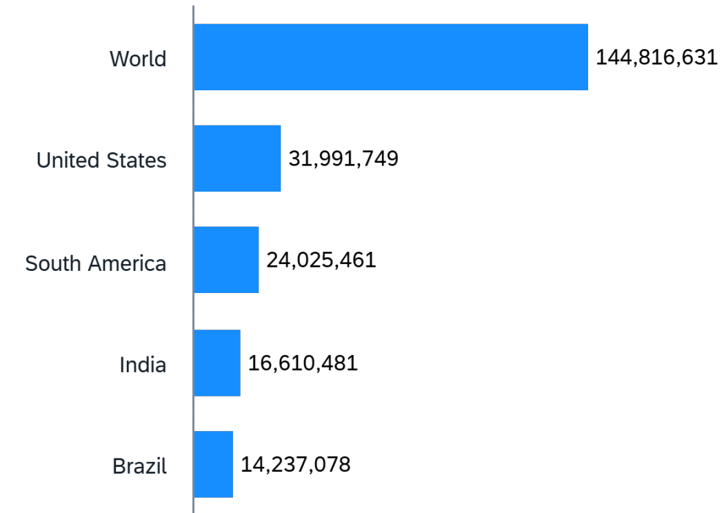
new_cases per date for Actual
